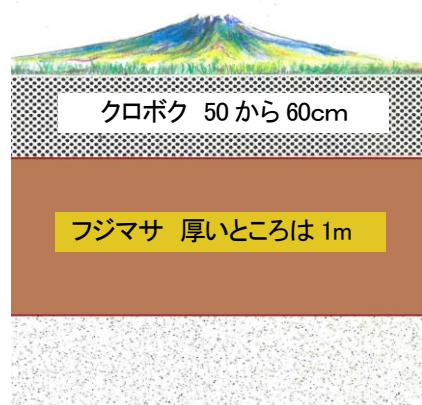
改良前の牧草地の地層イメージ
